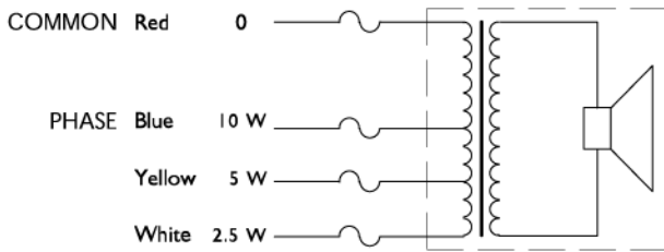
Принципиальная схема
