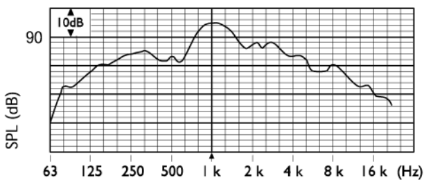
Частотная характеристика
