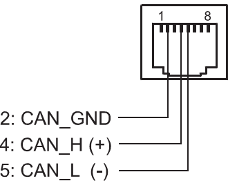
Рисунок 6.7: Назначение контактов порта CAN
