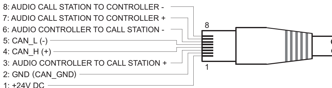
Рисунок 6.6: Назначение контактов разъема CST BUS
