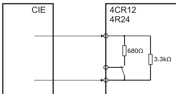
Рисунок 6.13: Внутренняя конфигурация контакта REL (VDE 0833-4)
