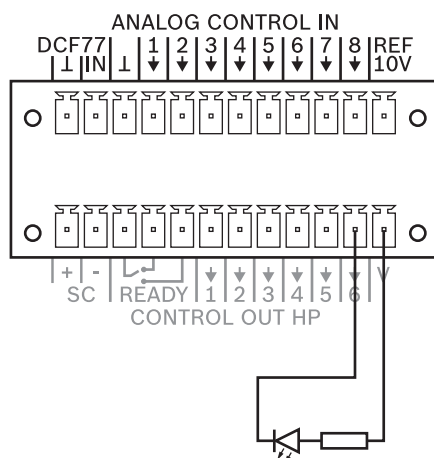
Рисунок 6.14: Пример использования выхода управления высокой мощности (светодиод с последовательным резистором)
