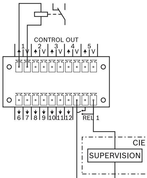
Рисунок 6.12: Подключение реле и контактов управления CIE к порту CONTROL OUT
