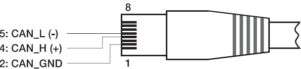
Рисунок 6.8: Назначение контактов разъема CAN
