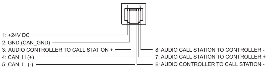
Рисунок 6.5: Назначение контактов порта CST BUS
