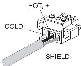
Рисунок 6.1: Сбалансированное подключение
