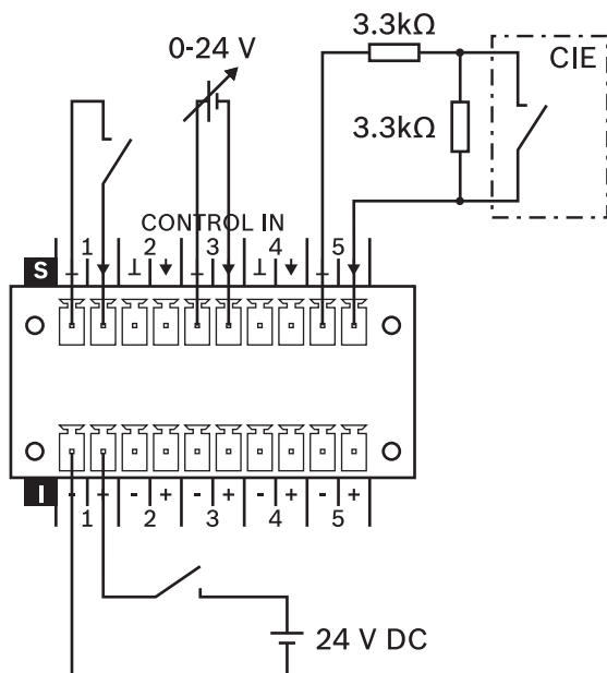
Рисунок 6.9: Использование контролируемых и изолированных входов порта CONTROL IN
