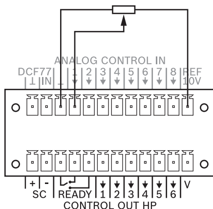
Рисунок 6.10: Пример использования управляющего входа при аналоговом входном сигнале
