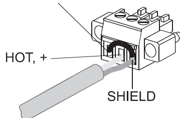
Рисунок 6.2: Несбалансированное подключение
