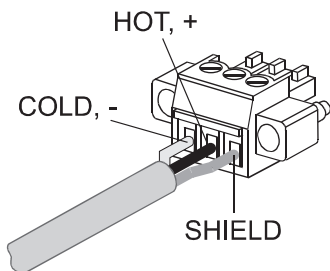
Рисунок 6.3: Сбалансированное подключение
