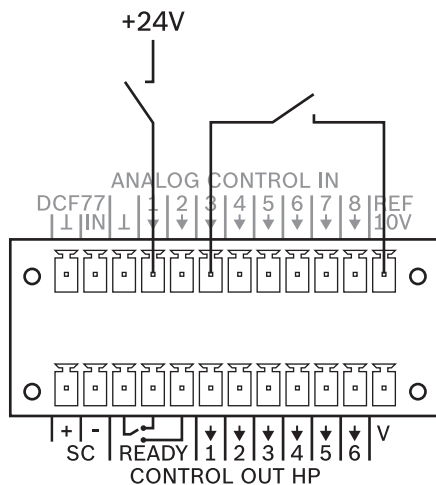
Рисунок 6.11: Пример использования управляющего входа при приеме двух цифровых выходных сигналов
